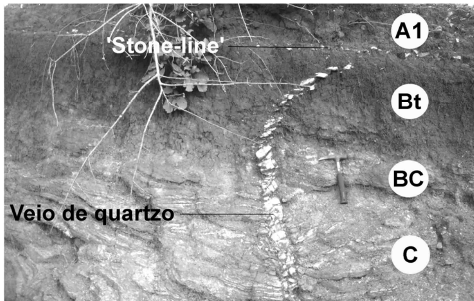
Figura 3 – Corte em um perfil vertical de Luvisolo crômico típico, localizado no terço superior de um interflúvio da superfície de piso semi-árida, ao sul de Canindé (Ceará). Trata-se de um solo evoluído tendo todas as características de uma pedogênese fersialítica : (1) forte liberação do ferro, refletida pela cor marrom avermelhada (5 YR 4/4 úmido) do horizonte Bt ; (2) quantidades importantes de minerais argilosos 2/1, confirmadas por análise DRX. A deformação do veio de quartzo se explica através da pedogênese do solo vermelho (remoção geoquímica e desaparecimento de matéria no entorno do quartzo resistente), talvez auxiliada por processos de rastejamento a partir do interflúvio de fraca declividade. Foto F. Bétard.
